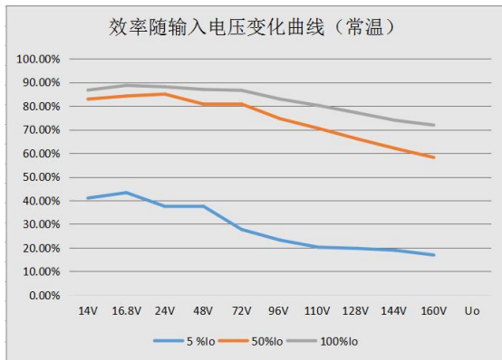
WLD10-H1D54(F/H)效率随输入电压变化曲线 (常温)
