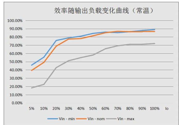
WLD10-H1D54(F/H)效率随输出负载变化曲线 (常温)
