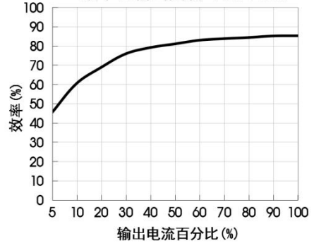
VSD3-B2415 效率Vs输出负载 (Vin=24V)
