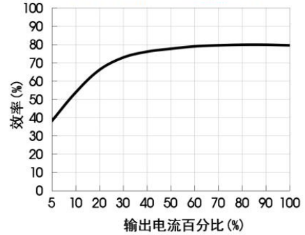
VSD3-B1205 效率 Vs 输出负载 (Vin=12V)
