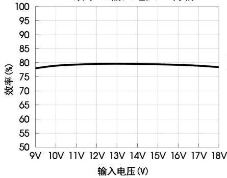
VSD3-B2415 效率Vs输入电压 (满载)
