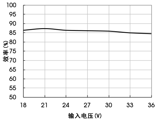
VP3-E2415 效率 Vs 输入电压 (满载)
