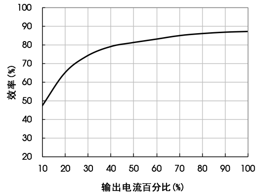
VP3-E2415 效率 Vs 输出负载 (标称输入)
