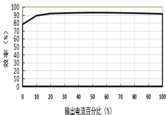
效率Vs输出负载 (Vin=48V)
