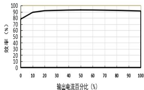
效率Vs输出负载 (Vin=48V)
