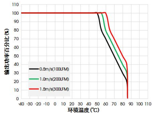
VOSB100-B48xxF 温度降额曲线
