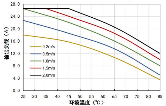
15VDC 输出 (无散热片) 温度降额曲线 (Vin=48V)
