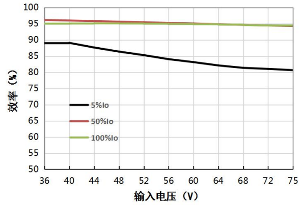
28VDC 输出 效率 VS 输入电压
