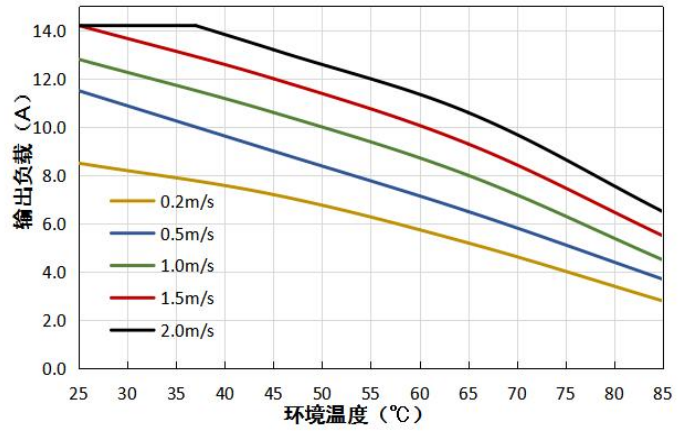
15VDC 输出 (带 H 散热片) 温度降额曲线 (Vin=48V)
