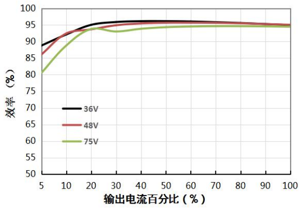
28VDC 输出 效率 VS 输出负载
