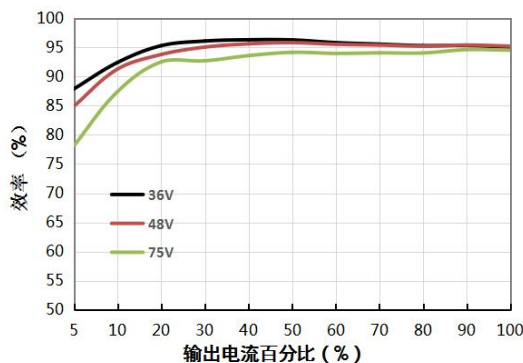
15VDC 输出 效率 VS 输出负载
