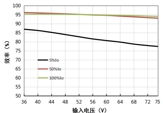
15VDC 输出 效率 VS 输入电压
