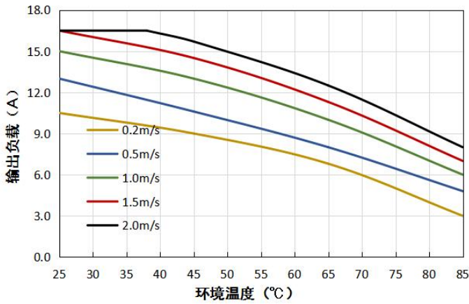
12VDC 输出 (带 H 散热片) 温度降额曲线 (Vin=48V)
