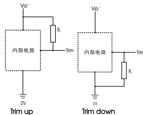
Trim 的使用电路(虚线框为产品内部)
