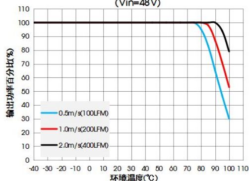
VOEB75-F4824FN 温度降额曲线 (Vin=48V)
