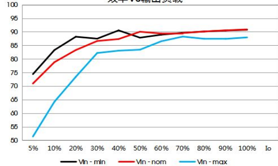
VOEB75-F4848(F)N 效率VS输出负载
