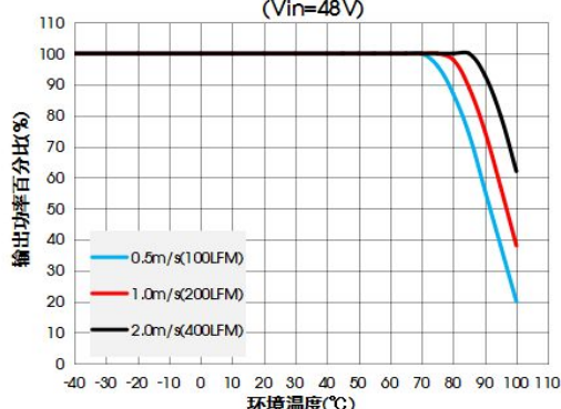
VOEB75-F4824N 温度降额曲线 (Vin=48V)
