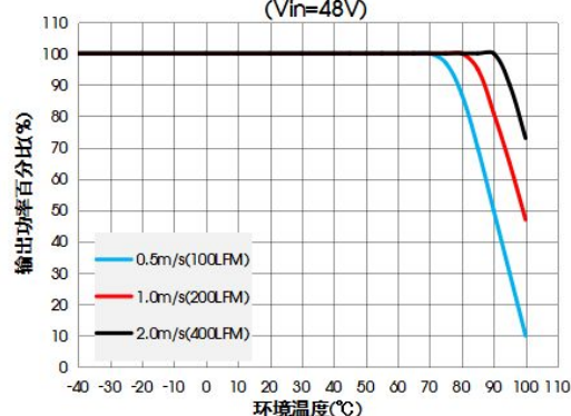
VOEB75-F4812FN 温度降额曲线 (Vin=48V)
