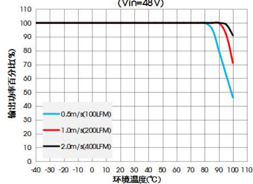
VOEB75-F4828FN 温度降额曲线 (Vin=48V)
