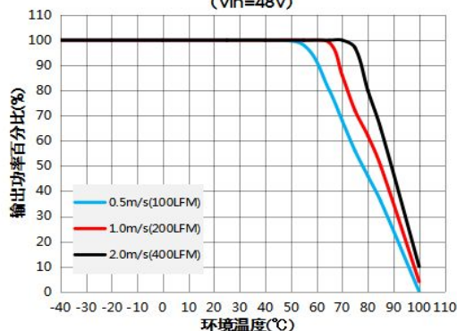
VOEB75-F4828N 温度降额曲线 (Vin=48V)
