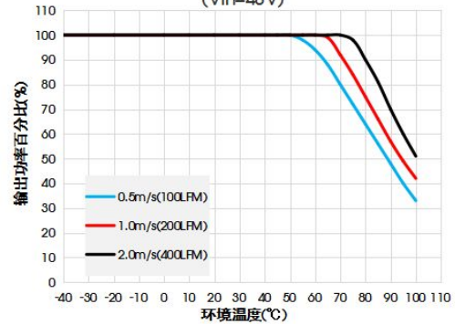
VOEB75-F4803FN 温度降额曲线 (Vin=48V)
