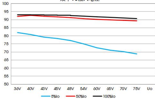
VOEB75-F4828(F)N 效率VS输入电压
