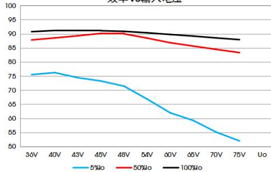
VOEB75-F4848(F)N 效率VS输入电压
