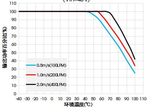
VOEB75-F4803N 温度降额曲线 (Vin=48V)
