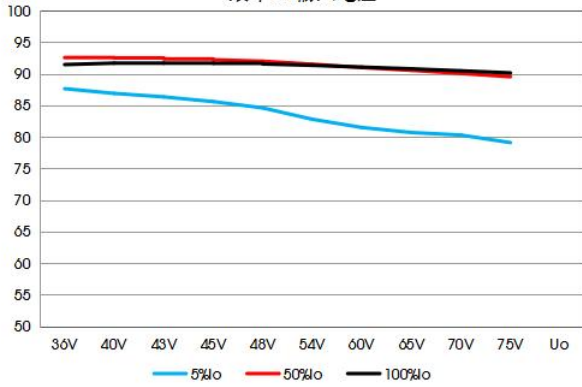
VOEB150-F4828(F)N 效率VS输入电压
