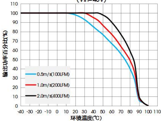
VOEB150-F4805N 温度降额曲线 (Vin=48V)
