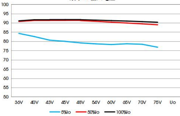
VOEB150-F4848(F)N 效率VS输入电压
