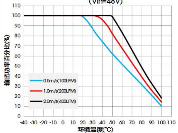
VOEB150-F4828FN 温度降额曲线 (Vin=48V)
