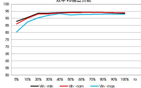
VOEB150-F4812(F)N 效率 VS 输出负载
