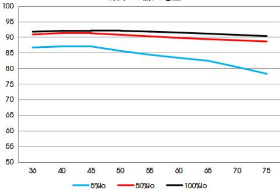
VOEB150-F4805N 温度降额曲线 (Vin=48V)
