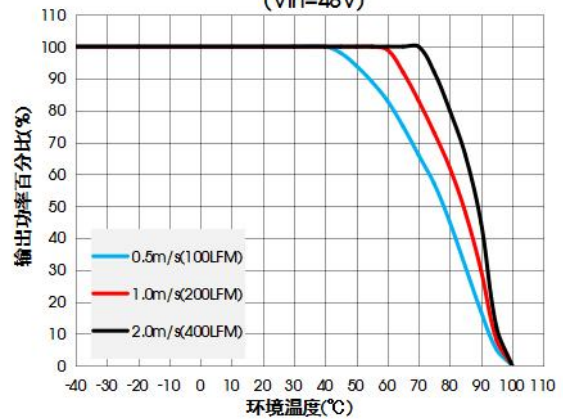
VOEB150-F4812FN 温度降额曲线 (Vin=48V)
