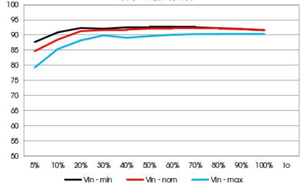
VOEB150-F4828(F)N 效率VS输出负载
