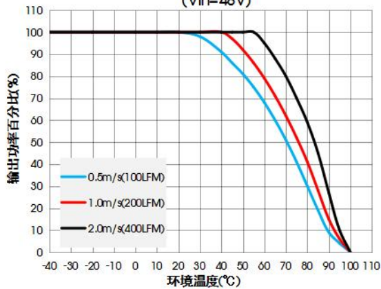
VOEB150-F4812N 温度降额曲线 (Vin=48V)
