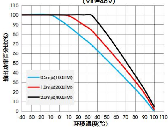
VOEB150-F4828N 温度降额曲线 (Vin=48V)
