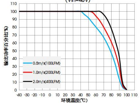
VOEB150-F4805FN 温度降额曲线 (Vin=48V)
