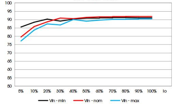
VOEB150-F4848(F)N 效率VS输出负载
