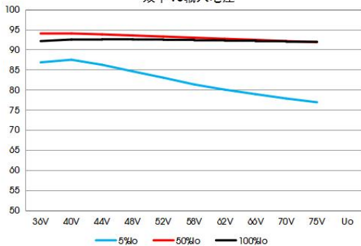
VOEB150-F4812(F)N 效率 VS 输入电压
