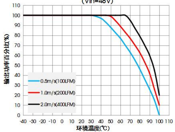
VOEB150-F4828FN 温度降额曲线 (Vin=48V)
