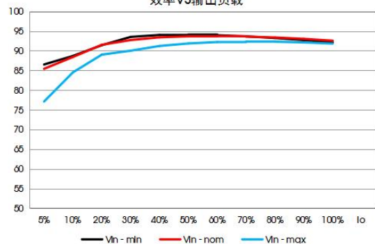
VOEB150-F4812(F)N 效率 VS 输出负载
