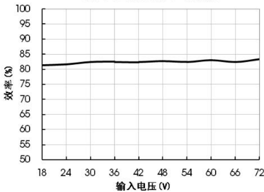
US3-D480512 效率Vs输入电压 (满载)
