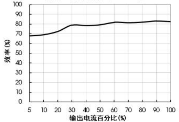
US3-D480512 效率Vs输出负载 (Vin=48V)
