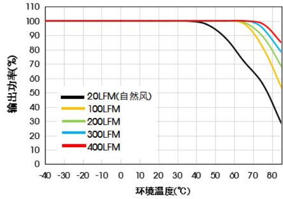
UQB100-F2424F 温度降额曲线图 (Vin=24V)
