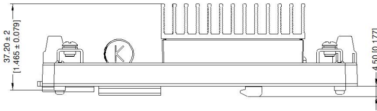
前视图
