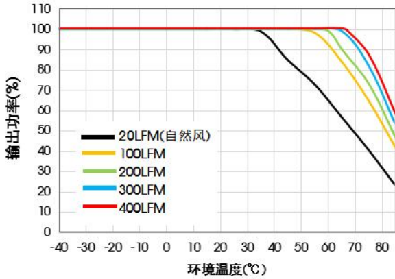
UQB100-F2424 温度降额曲线图 (Vin=24V)
