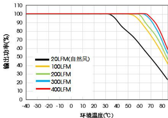
UQB100-F2424 温度降额曲线图 (Vin=24V)
