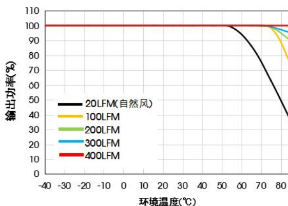
UQB100-F2424H 温度降额曲线图 (Vin=24V)
