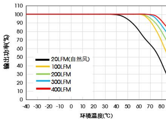
UQB100-F2424F 温度降额曲线图 (Vin=24V)
