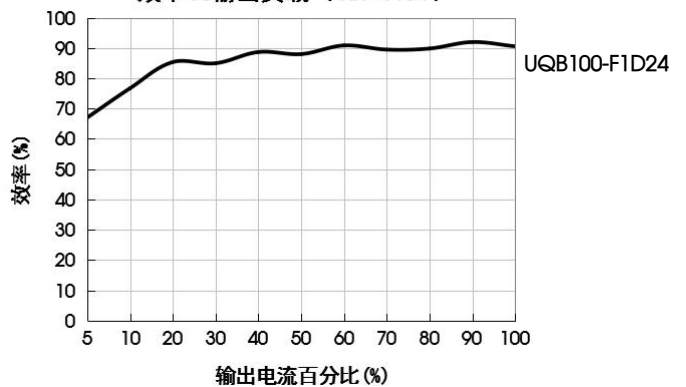
效率Vs输出负载 (Vin=110V)
