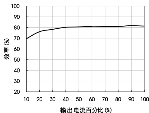
UP6-H4815 效率Vs输出负载 (标称输入)
