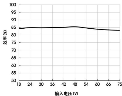
效率Vs输入电压 (满载)
