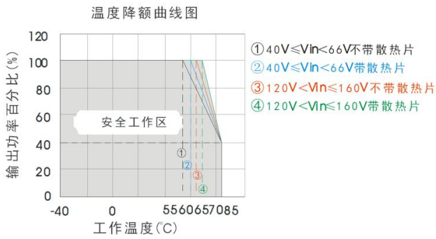
5VDC 输出 图 1
