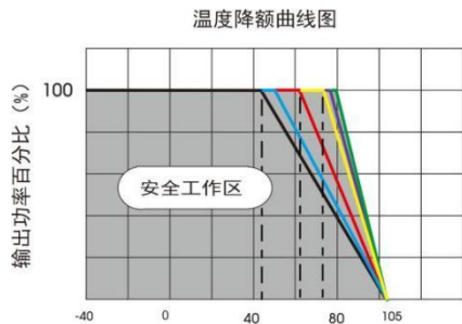
UHB150-F1D05H 温度降额曲线(Vin=110V)
