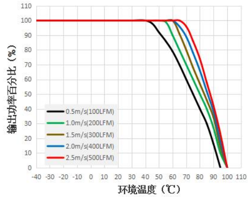
UFB400-F1D12H 温度降额曲线图
