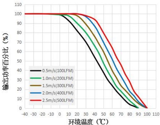
UFB400-F1D24 温度降额曲线图
