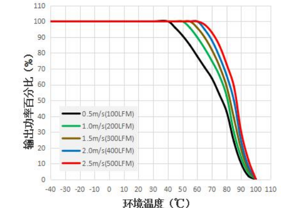
UFB400-F1D54H 温度降额曲线图
