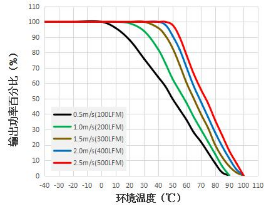
UFB400-F1D54 温度降额曲线图
