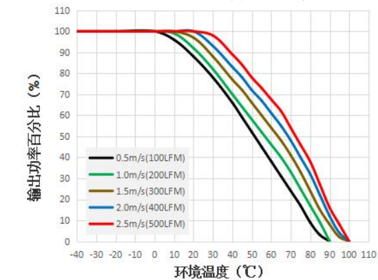
UFB400-F1D54 温度降额曲线图
