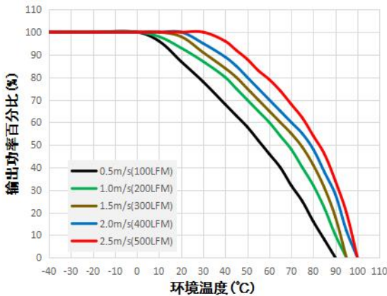
UFB400-F1D05 温度降额曲线图
