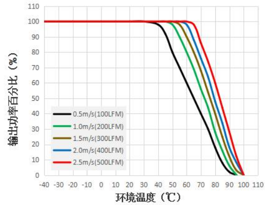
UFB400-F1D36H 温度降额曲线图
