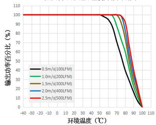
UFB400-F1D15H 温度降额曲线图
