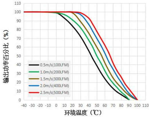
UFB400-F1D36 温度降额曲线图
