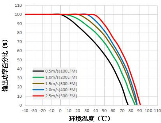
UFB400-F1D48 温度降额曲线图
