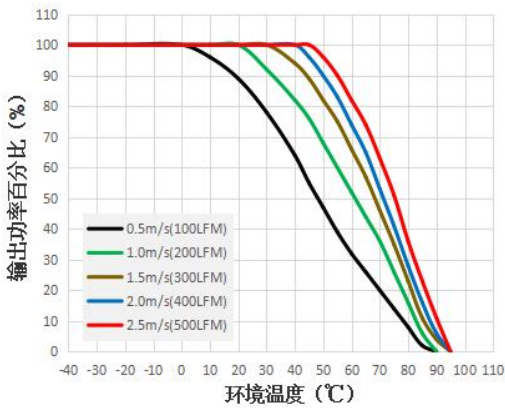
UFB400-F1D15 温度降额曲线图
