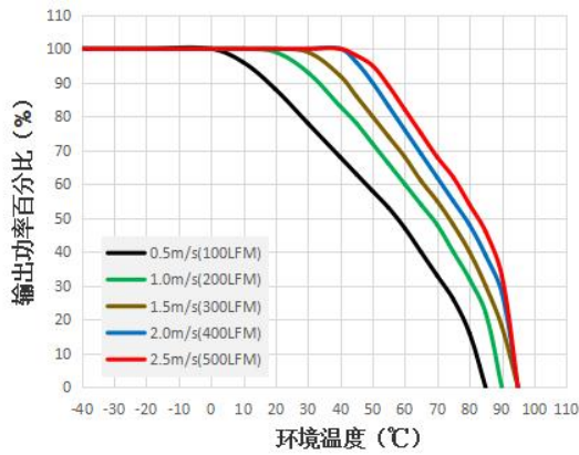
UFB400-F1D12 温度降额曲线图
