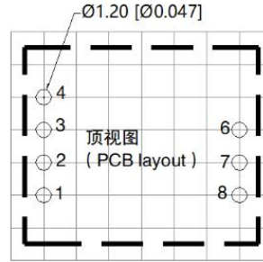
引脚方式
