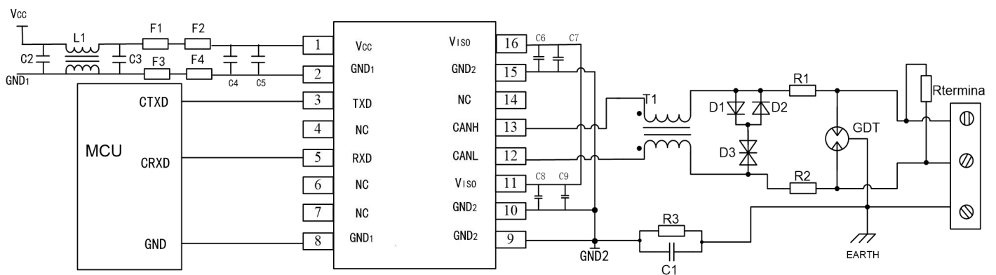
图 9.端口保护推荐电路
