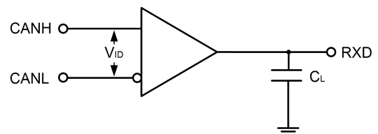
图 2. 接收器测试电路
