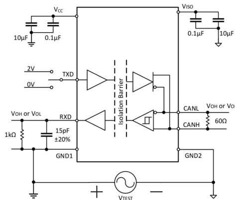
图 6.CMTI 测试电路
