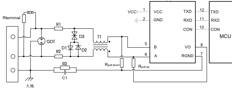
图 2. 端口保护推荐电路
