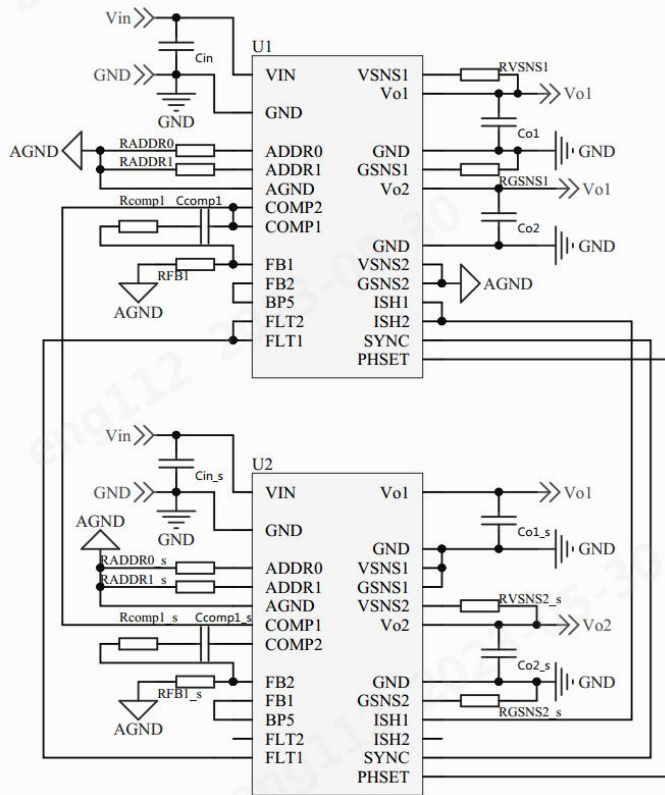
三相应用
