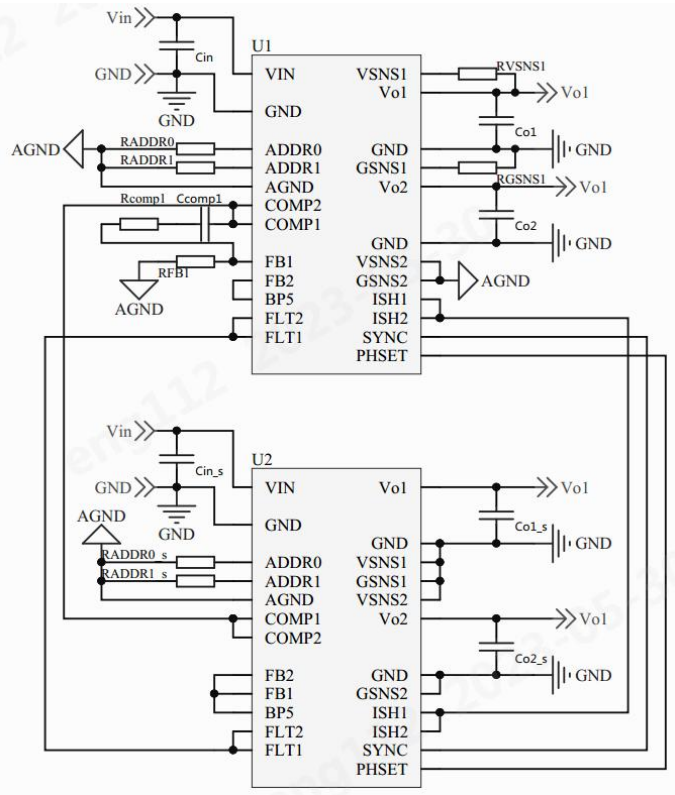
四相应用
