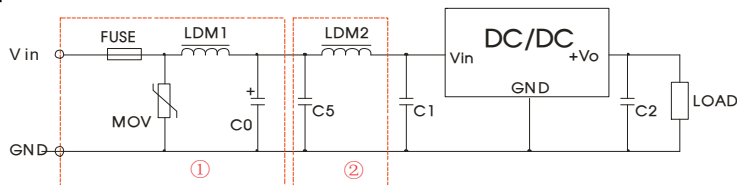
图 3：推荐电路
