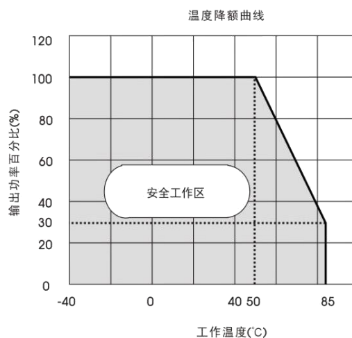
图2 KS0.3-78U24(L) ( V_{in}\geq 60V )
