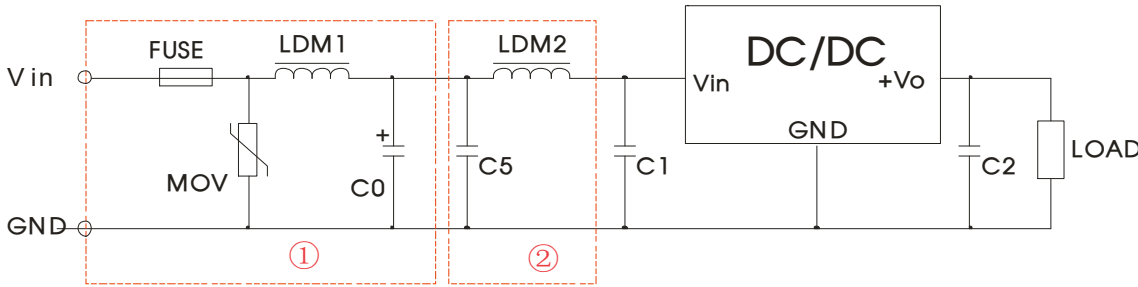
图 4 EMC 推荐电路
