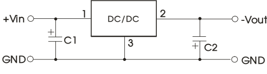
负输出应用电路
