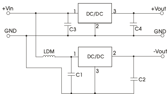
图 3 正负输出并联应用电路
