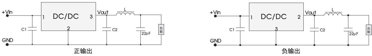
图 4 “LC”滤波应用电路
