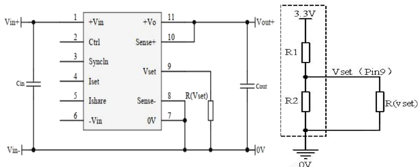
图 5 Vset 外接调整电阻接线图
