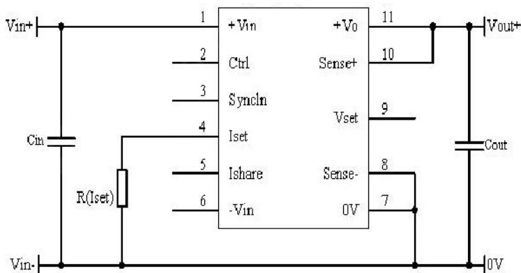
图 9 Iset 外接调整电阻接线图
