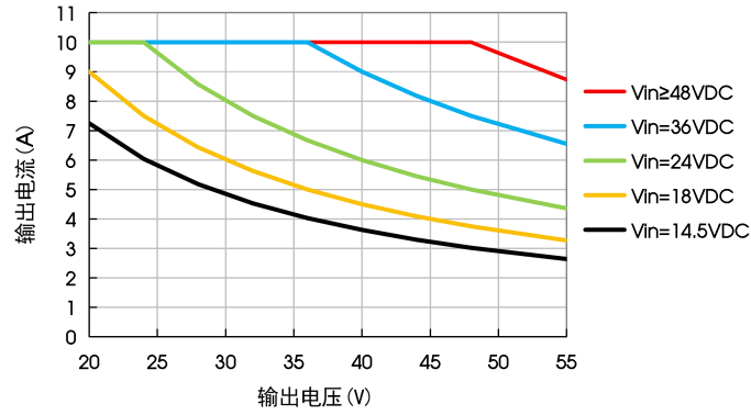
KEB10-UB48xx(F) 输出电流降额曲线
