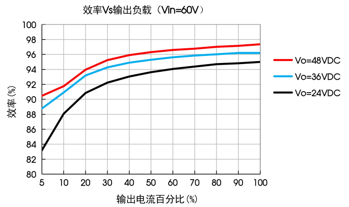
KEB10-UB4848(F)
