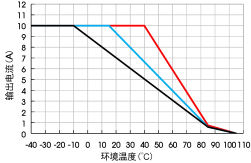
KEB10-UB6048 温度降额曲线 (Vin=60V, Vo=24V)
