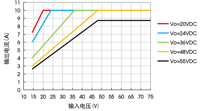
KEB10-UB4848(F) 输出电流降额曲线
