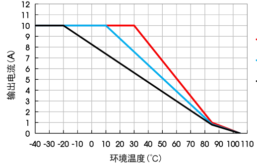
KEB10-UB6048 温度降额曲线 (Vin=60V, Vo=36V)
