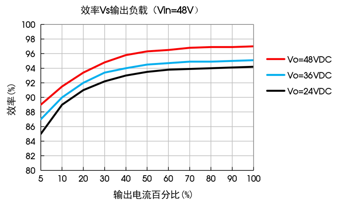
KEB10-UB4848(F)
