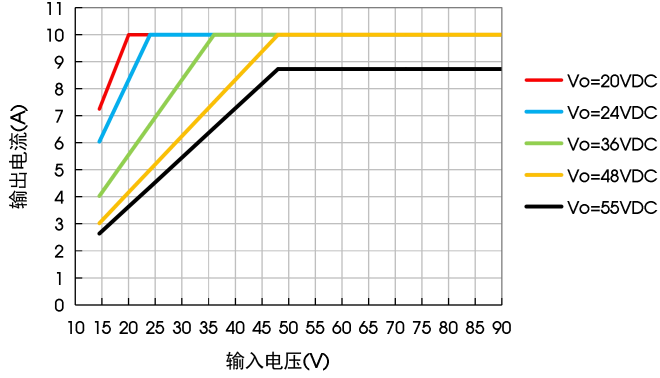
KEB10-UB6048(F) 输出电流降额曲线
