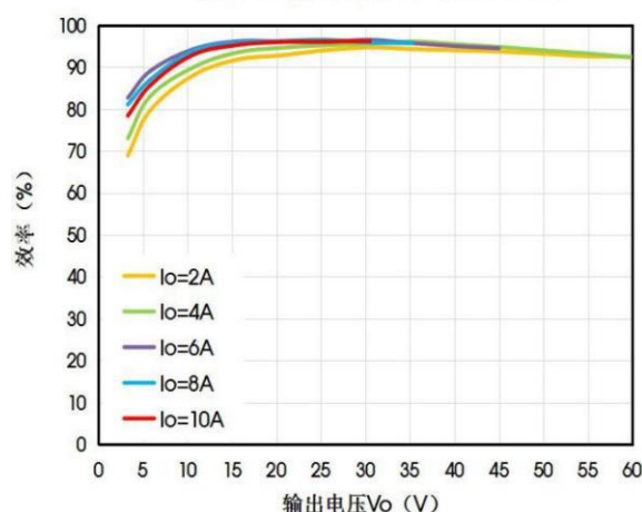
效率VS输出电压Vo (Vin=60V)
