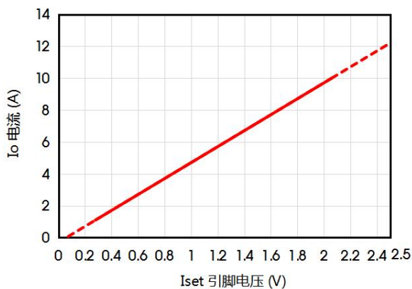
Iset 引脚电压 VS Io 电流
