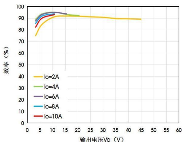
效率VS输出电压Vo (Vin=48V)
