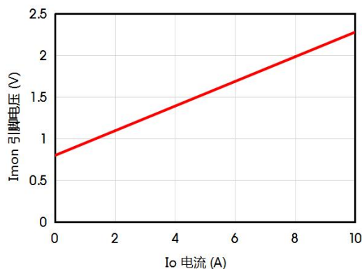
Io 电流 VS Imon 引脚电压
