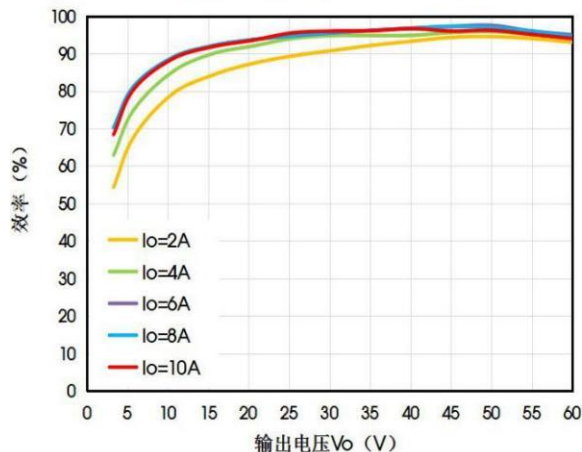
效率VS输出电压Vo (Vin=60V)
