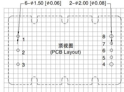
引脚方式
