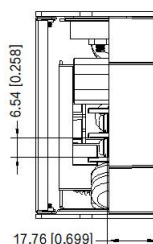
右视图
