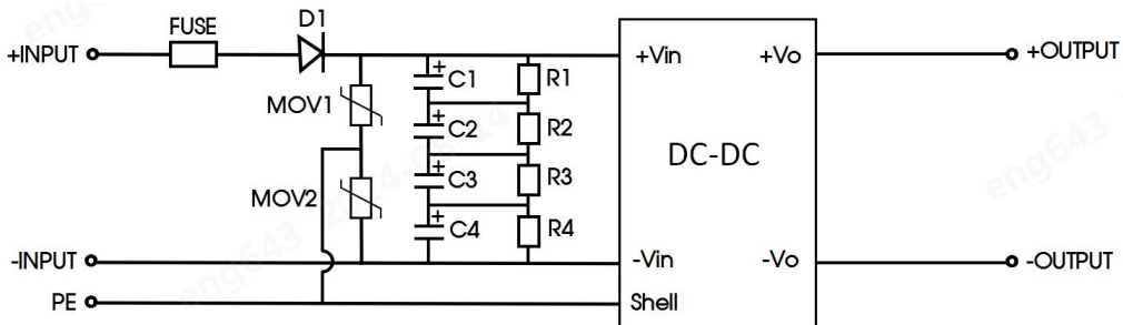
图 2: 推荐电路
