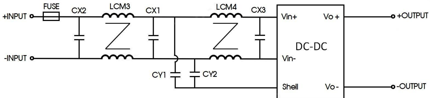
图 3: CLASS II 推荐电路
