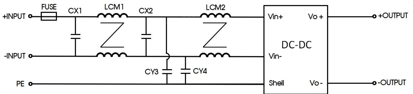
图 2: CLASS I 推荐电路
