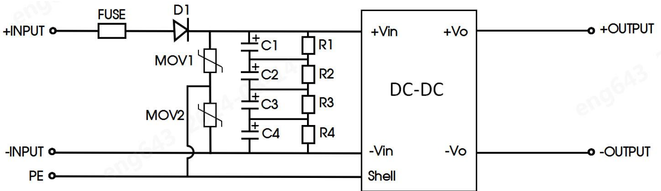
图 2: 推荐电路
