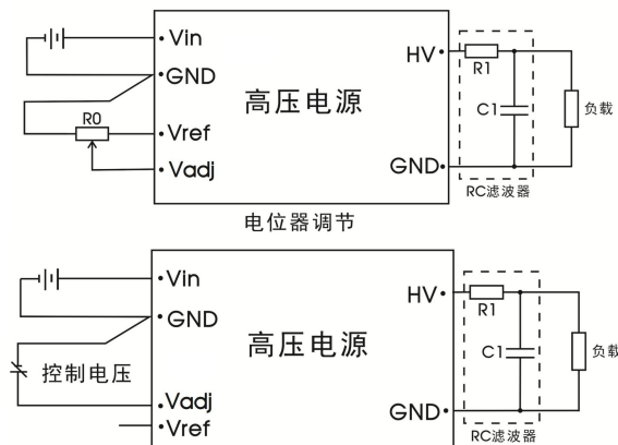
图2 输出电压外部调节方式
