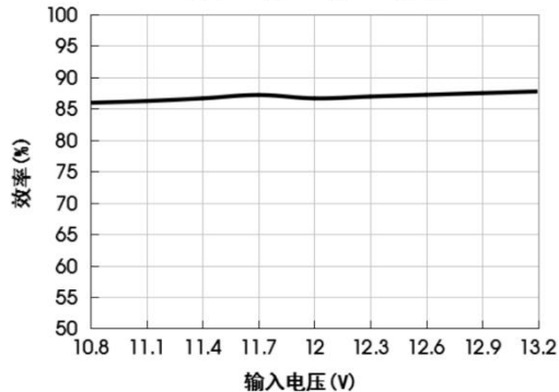
DXT2-B1205 效率Vs输入电压 (满载)
