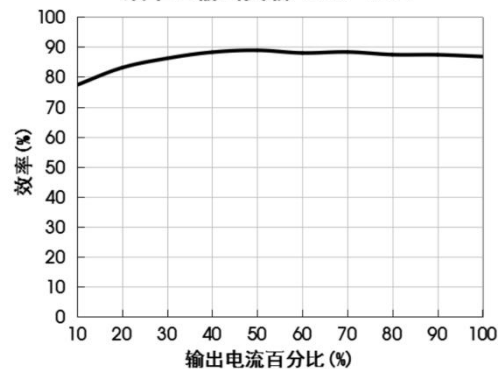
DXT2-B1205 效率Vs输出负载 (Vin=12V)
