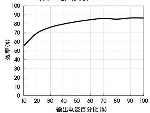
DXT2-B2405 效率Vs输出负载 (Vin=24V)
