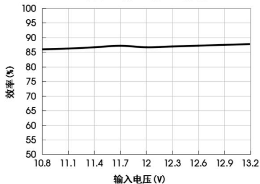
DXT2-B2405 效率Vs输入电压（满载）
