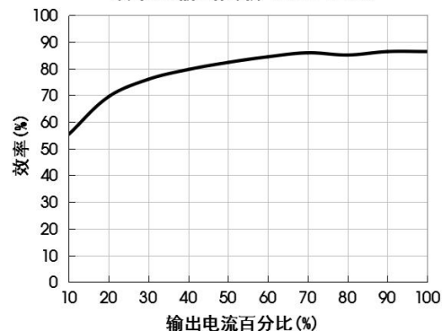
DXT2-B2405 效率Vs输出负载（Vin=24V）
