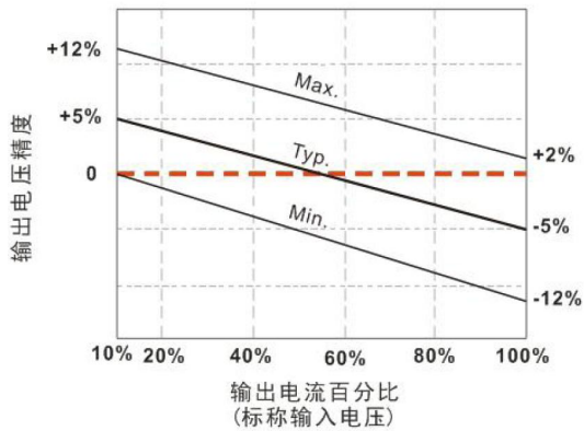
5VDC 输入, 3.3VDC 输出 误差包络曲线图
