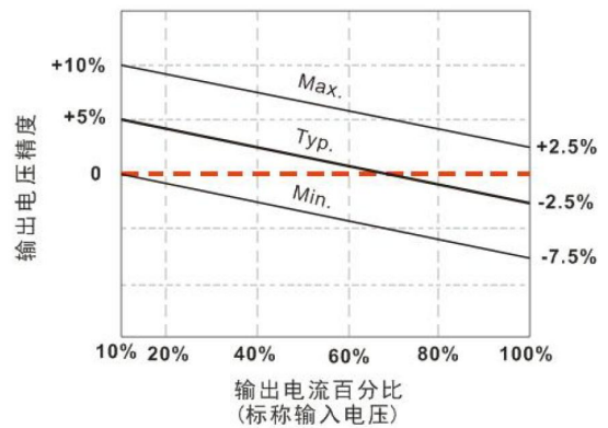
5VDC 输入, 其他输出 误差包络曲线图
