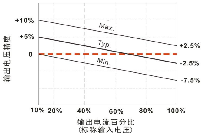
5VDC 输入 其他输出 误差包络曲线图
