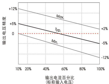
3.3VDC 输出
