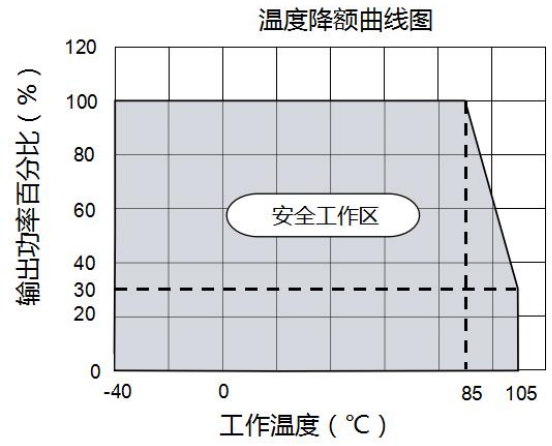
12/24V 输入 (DCS1-IH2405 除外)
