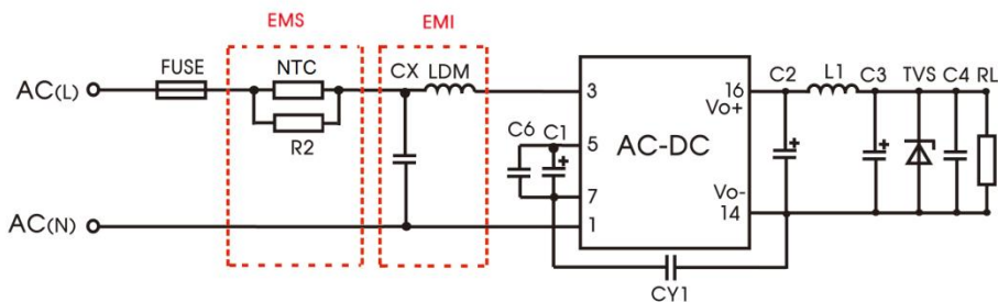
推荐电路 1
