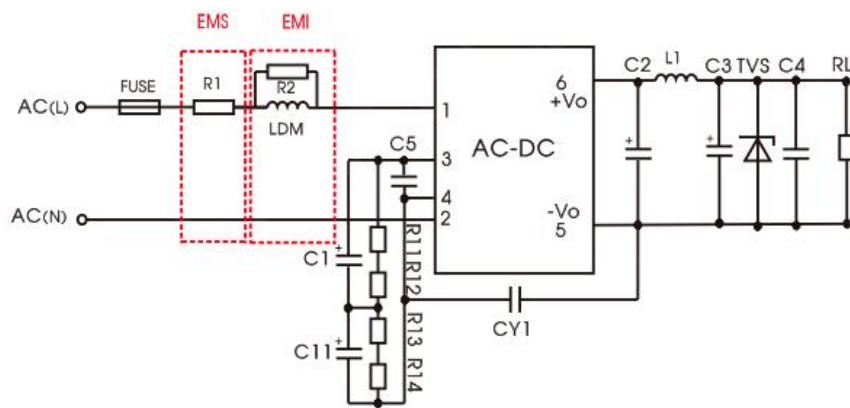
推荐电路 1
