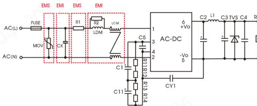
推荐电路 3
