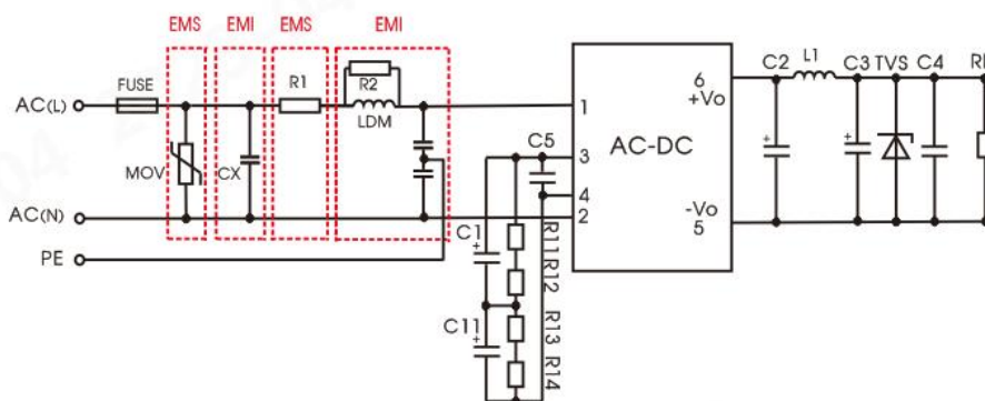
推荐电路 5
