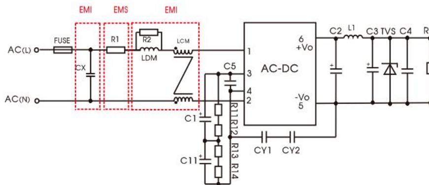
推荐电路 2
