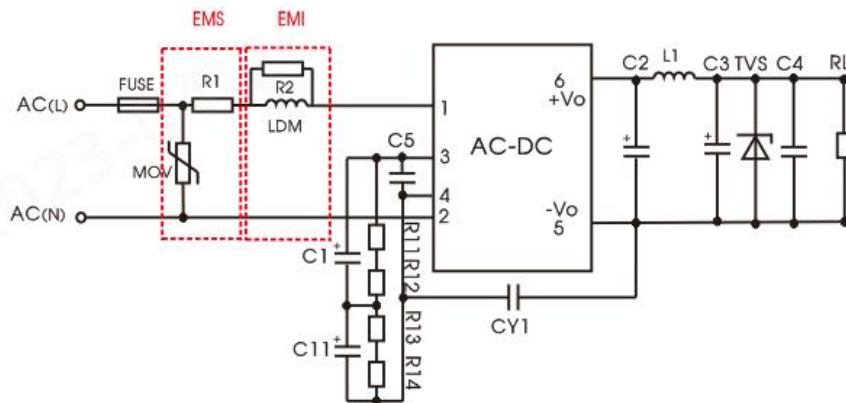
推荐电路 4
