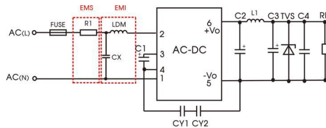
推荐电路 2
