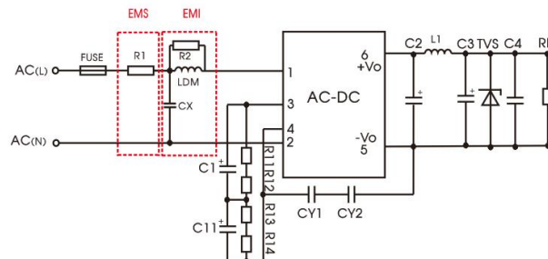
推荐电路 2
