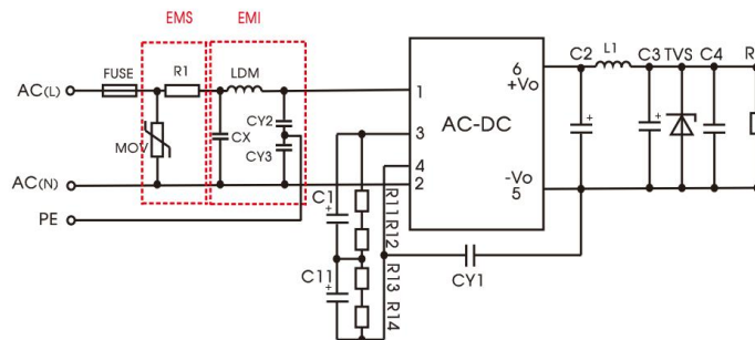
推荐电路 5
