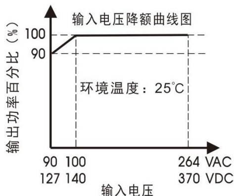
AOF350-Bxx-C 输入电压降额
