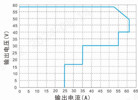
图1 输出外特性曲线*
