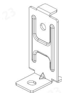
客选配件支架（PAA-069）
