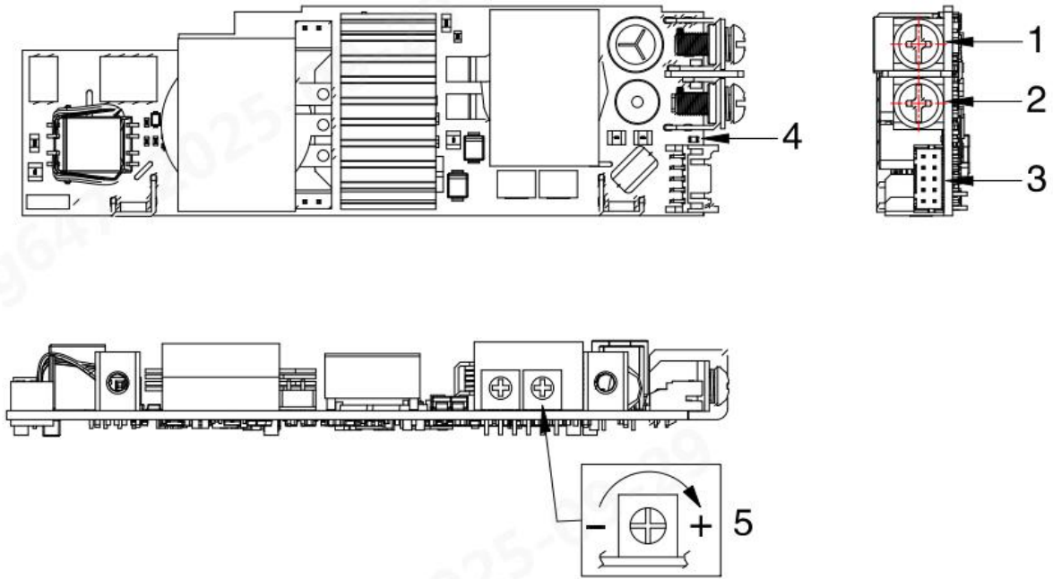
图 2：模块 AOP300-Bxx 外观信息
