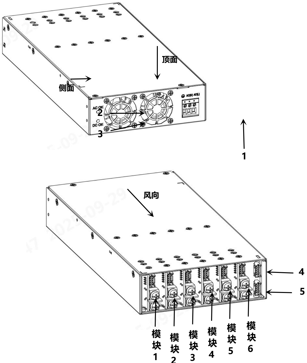
图 1: AMP1200-xxxxxx-xx 外观信息
