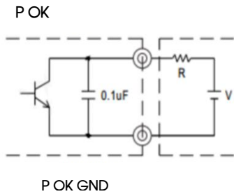
图 1 电源正常的内部回路（集电极开路的方法） (最大吸入电流 10mA, 最大电压 30V)
