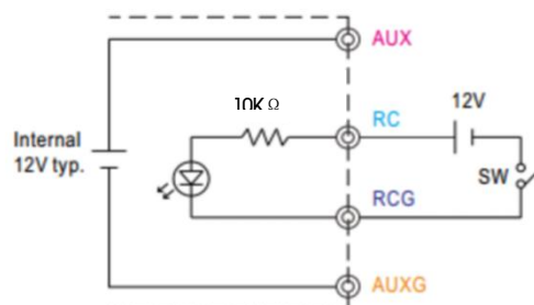
图 1 用外部电压
