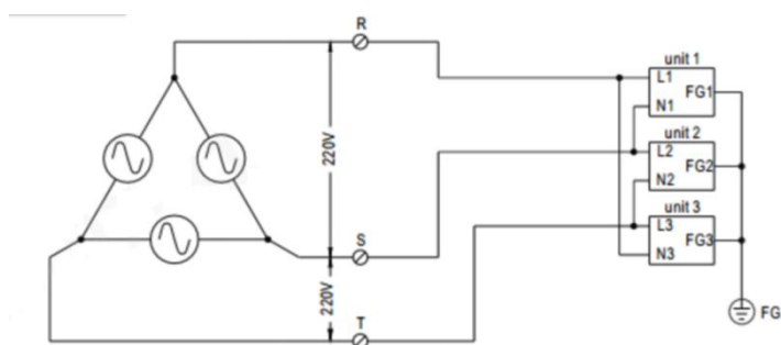
图 1 三相三线 220VAC 系统
