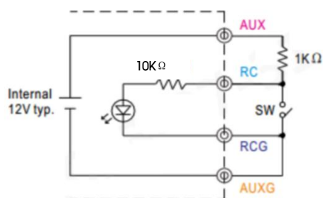
图 3 用内部 12V 辅助输出
