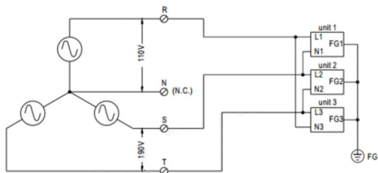
图 3 三相四线 190/110VAC 系统
