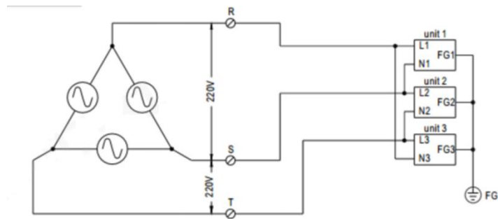
图 1 三相三线 220VAC 系统
